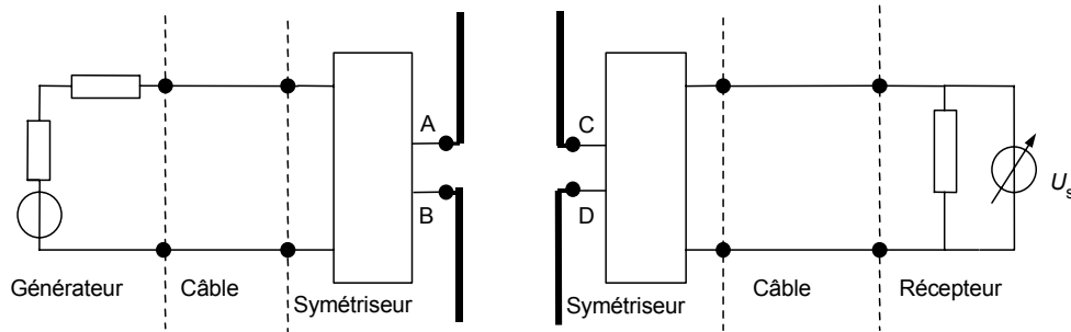
Figure 4 – Détermination de U_s(f) avec les antennes filaires dans leur position spécifiée
